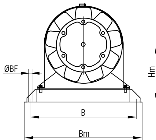
Support de chemise de refroidissement/moteur
