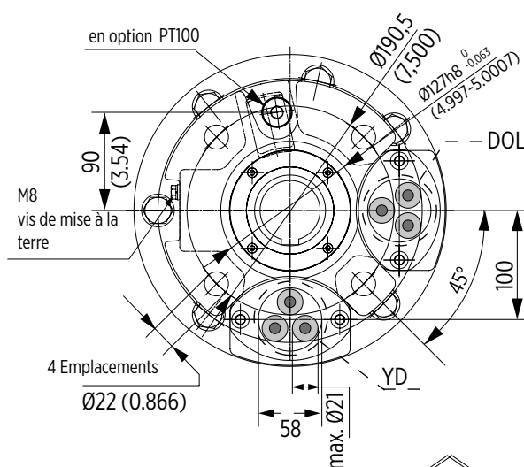
Cloche d'extrémité, supérieure
