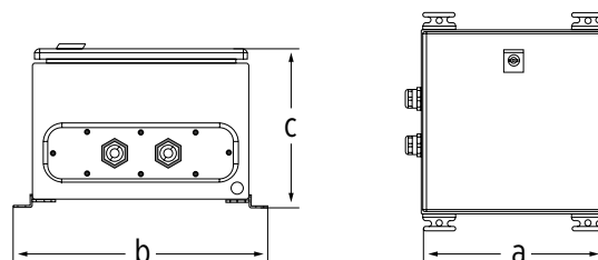
Filtres IP54 pour montage mural
