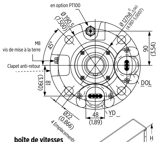
Cloche d'extrémité, supérieure
