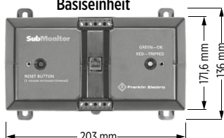
Basiseinheit
