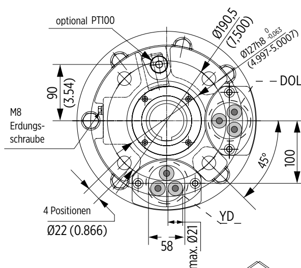
Oberes Lagerschild
