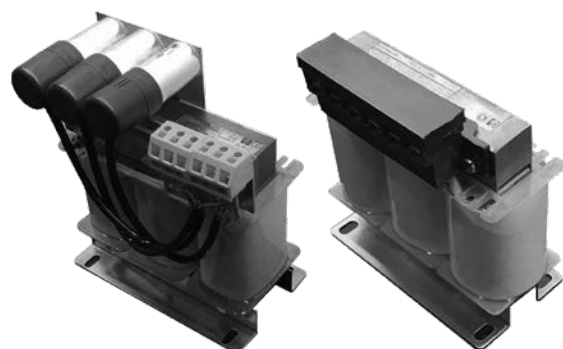
Sinus Ausgangsfiler
