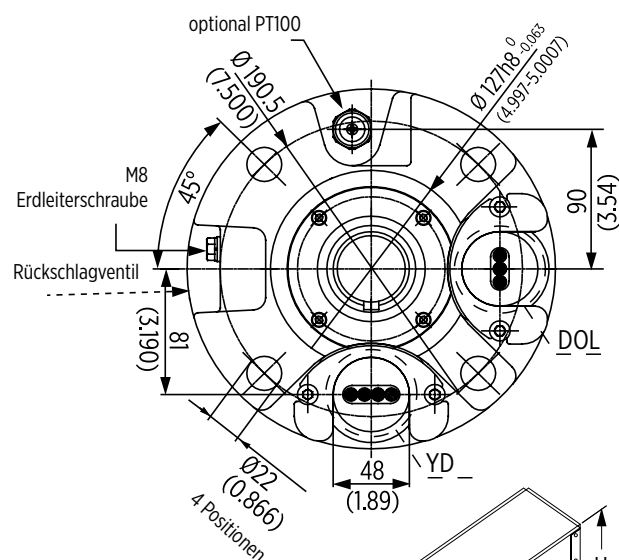
Motorbox
