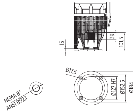
8"-MOTOR
