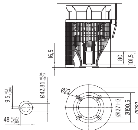
10"-MOTOR
